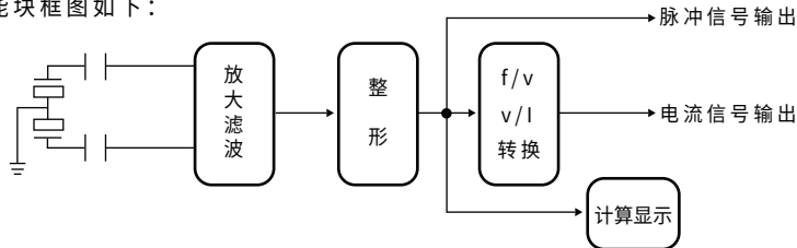
图2 流量计原理框图
