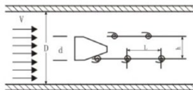
图1 旋涡形成示意图
