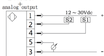
2 × NPN
